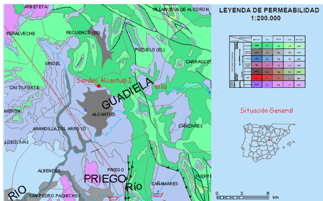
Figura 24. Mapa de permeabilidades de la UH 03.02.
