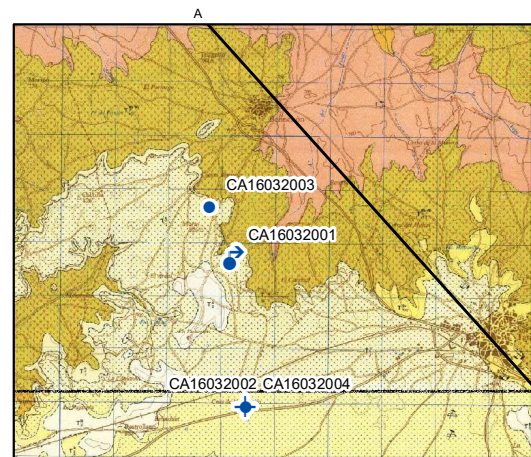
Escala 1:100.000 0 1 2 4 km
