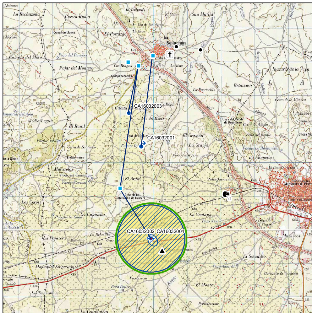
Escala 1: 50.000 0 0.5 1 2 km
