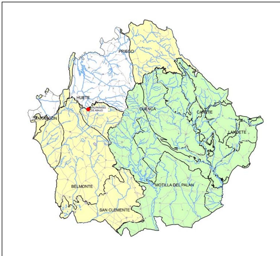
Figura 1. Ubicación de la localidad de Valparaíso de Abajo y del manantial (Coord. UTM 0530115-4435714).
