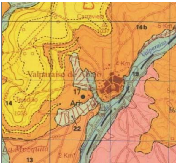
Figura 2. Encuadre Geológico. Hoja 608 “Huete” Serie MAGNA 1:50.000.
