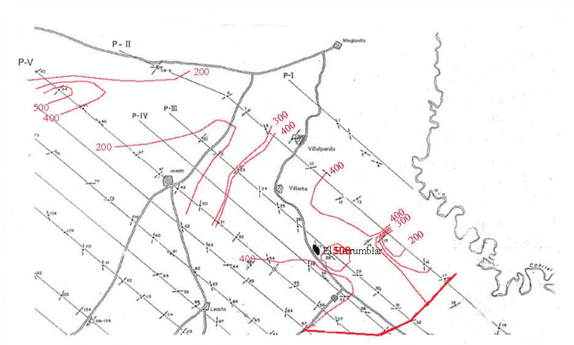
Figura 6.- Mapa de isohipsas del sustrato mesozoico. En rojo las profundidades desde la superficie.
