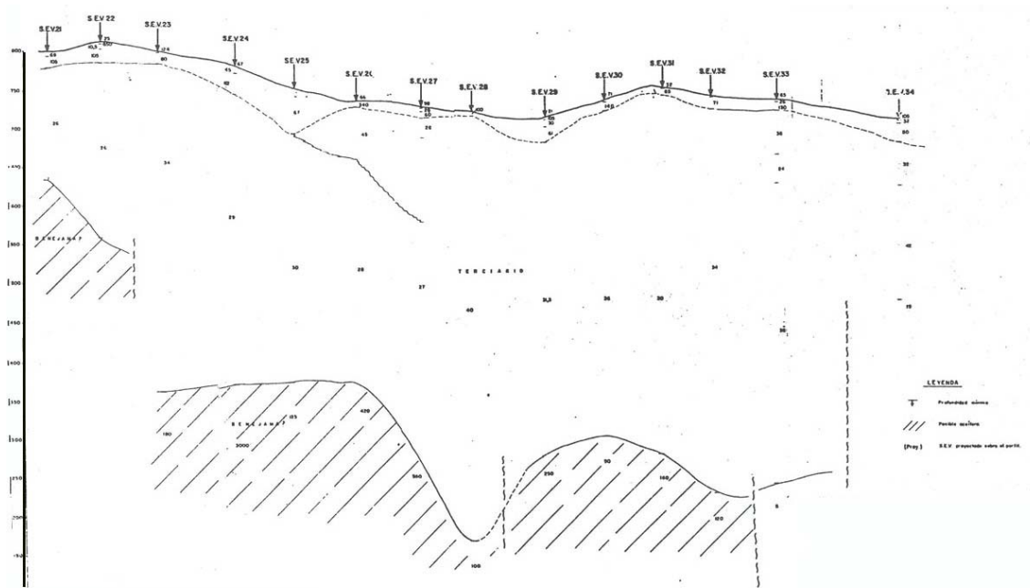
Figura 4. Perfil P III (IGME, 1984).
