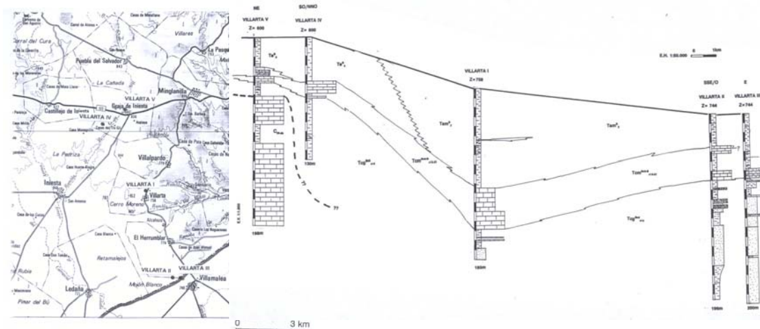
Figura 1.- Ubicación de los sondeos de investigación rerealizados para Villarta (IGME, 1998)
