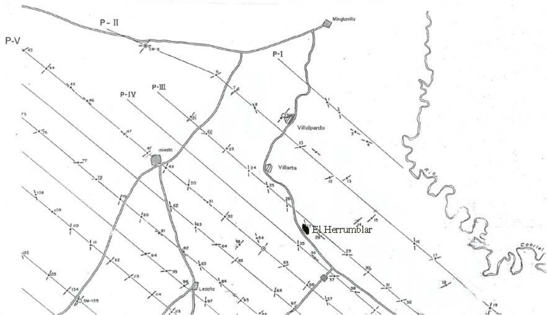
Figura 2.- Situación de los perfiles geoelectricos.
