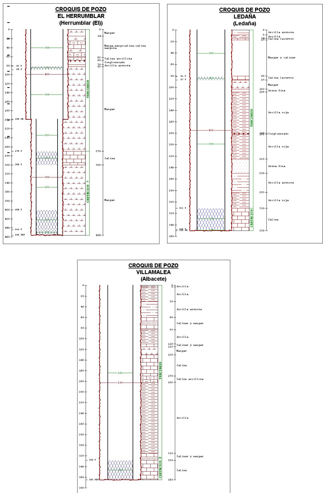
Figura 7.- Croquis de los sondeos de investigación realizados en El Herrumblar (IRYDA), Ledaña y Villamalea
