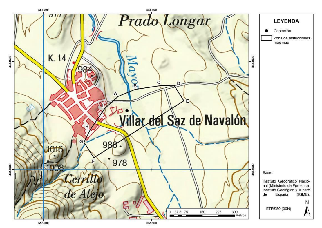
Figura 12. Sondeo de abastecimiento a Villar del Saz de Navalón y zona de restricciones máximas del perímetro de protección
