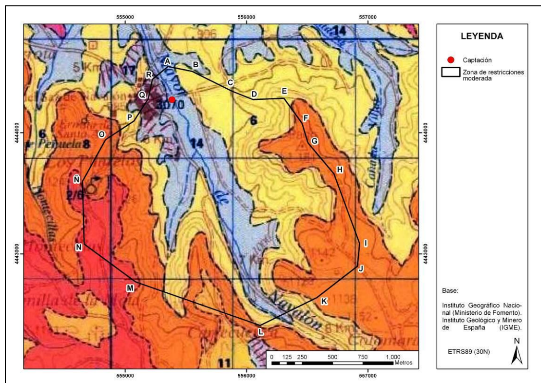
Figura 13. Sondeo de abastecimiento a Villar del Saz de Navalón y zona de restricciones moderada del perímetro de protección.
