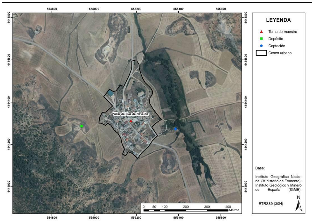
Figura 2. Sistema de abastecimiento del núcleo de Villar del Saz de Navalón.
