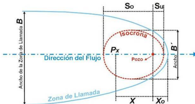
Figura 10. Método de Wyssling para el cálculo del tiempo de tránsito
