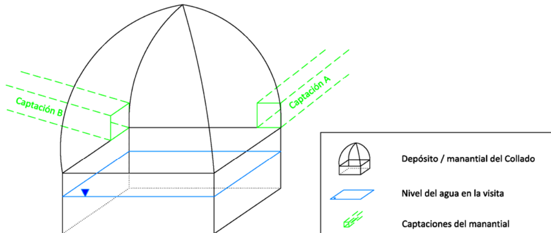
Figura 19. Esquema representativo del manantial / depósito de la Fuente del Collado.
