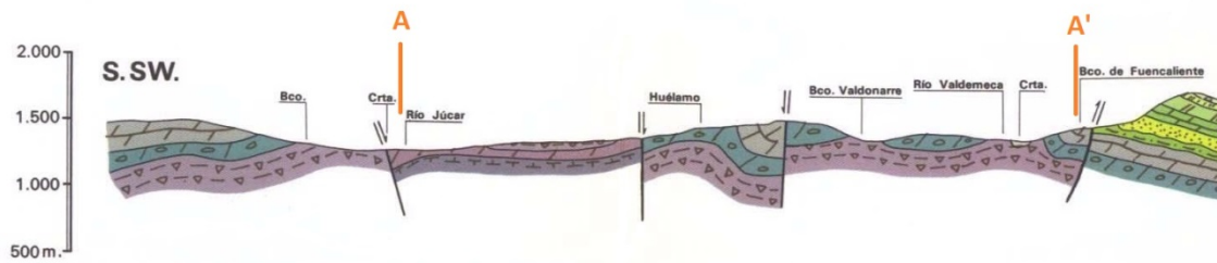
Figura 3. Corte geológico I-I' donde aparece el perfil A-A' a su paso por Huélamo (fuente: IGME, Mapa Geológico MAGNA 1:50.000, hoja nº 588-Zafrilla).
