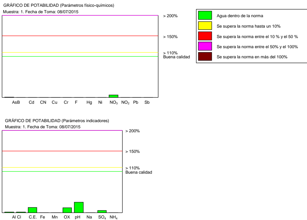
Figura 16. Gráfico de Potabilidad.
