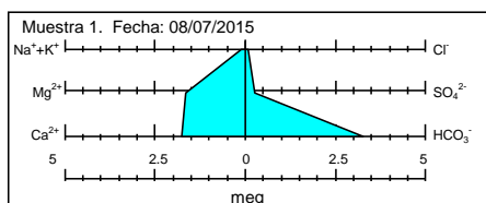
Figura 14. Diagrama de Stiff.
