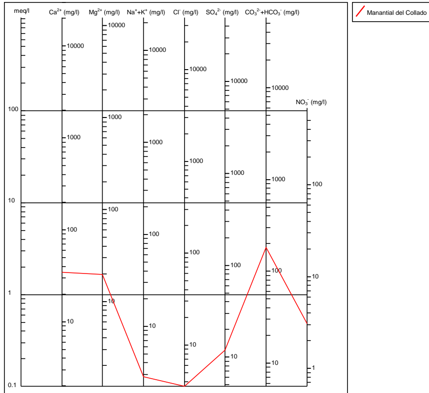
Figura 15. Diagrama de Schoeller.
