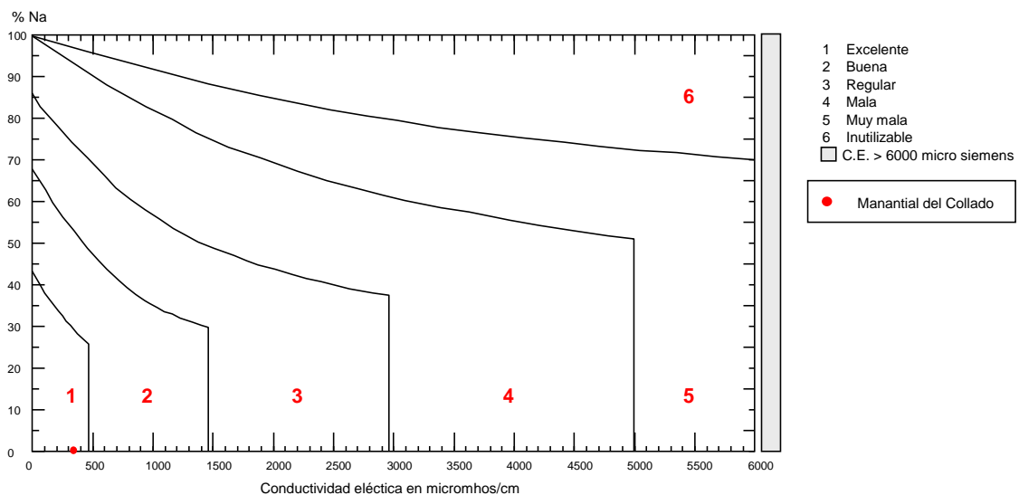
Figura 18. Diagrama de aptitud agrícola.
