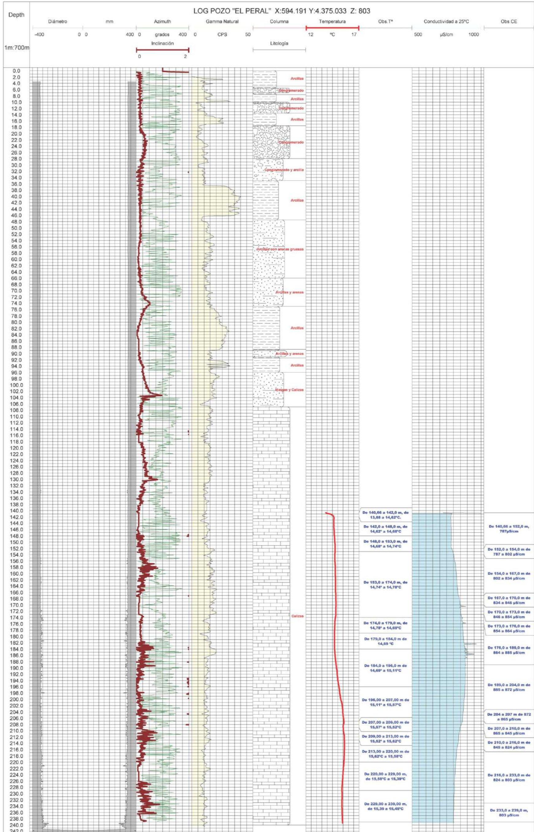
Figura 15.- Logs del sondeo "Pozo El Peral" Reconocido.
