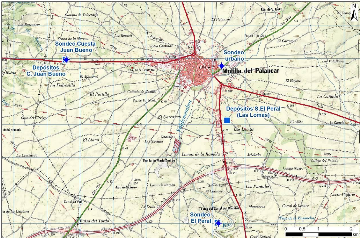
Figura 6. Elementos del sistema de abastecimiento sobre MTN E: 1/50.000
