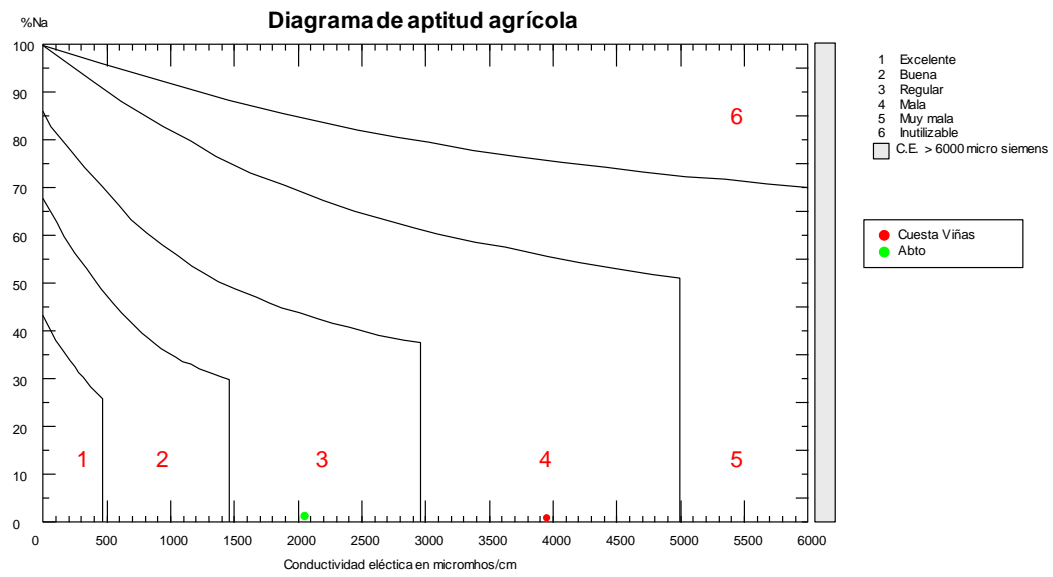
Figura 11. Diagrama de aptitud agrícola de ambas muestras
