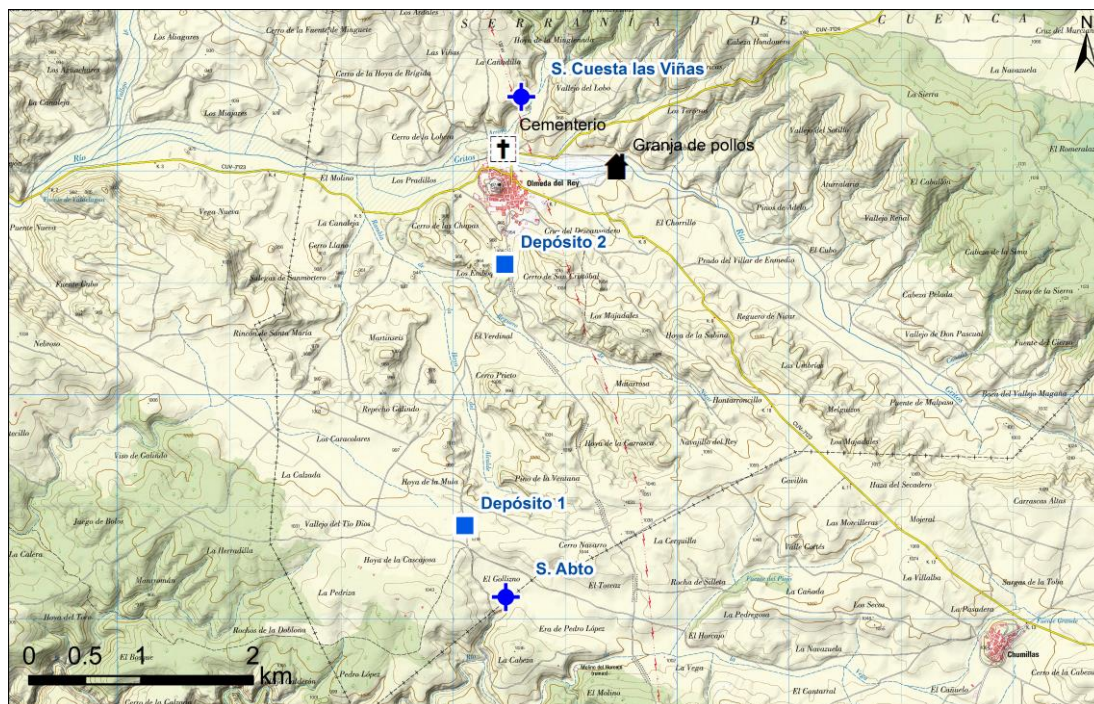
Figura 16. Focos potenciales de contaminación de los alrededores de Olmeda del Rey
