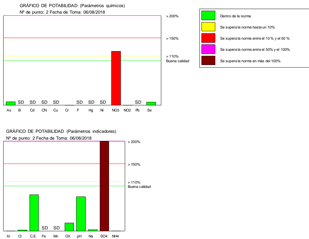
Figura 14. Gráficos de potabilidad del agua de Sondeo de abastecimiento
