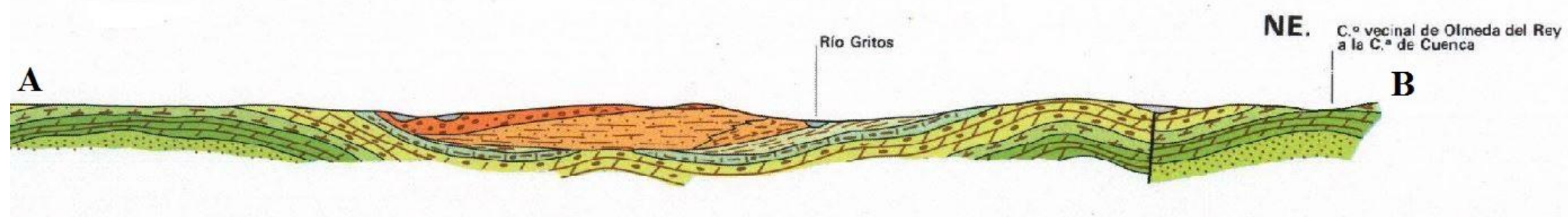
Figura 7. Mapa geológico y corte de los alrededores de Olmeda del Rey y ubicación de las captaciones. (Modificado de MAGNA 663)
