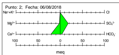
Figura 10. Diagramas de Stiff del sondeo de abastecimiento
