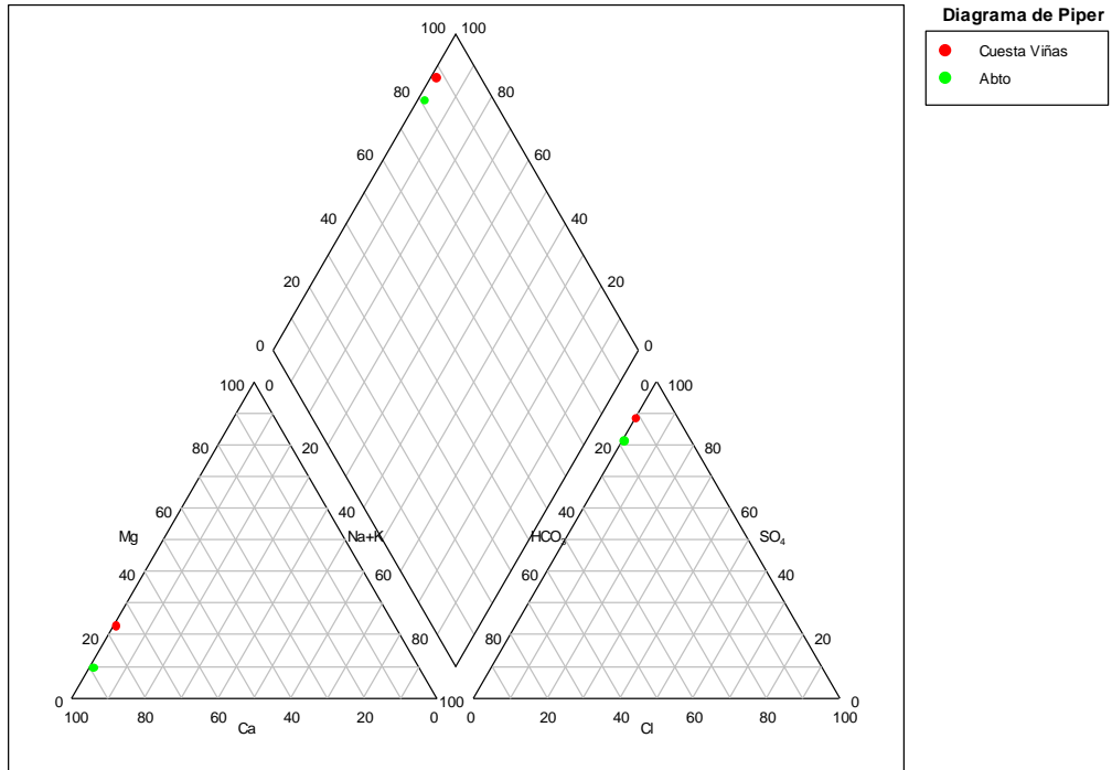
Figura 8. Diagrama de Piper-Hill-Langelier de ambos sondeos
