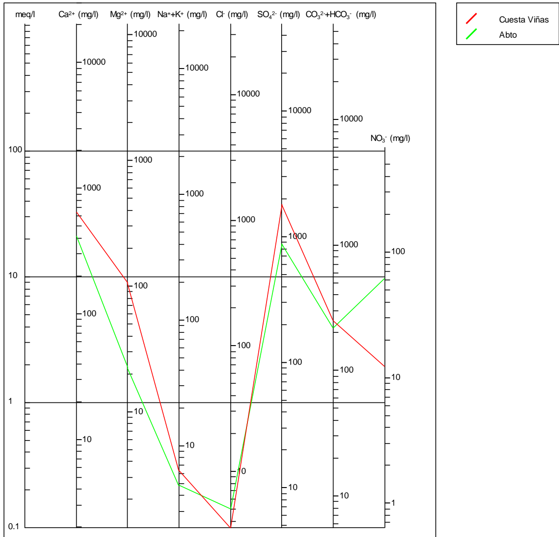
Figura 12. Diagrama de Schöeller de ambas muestras
