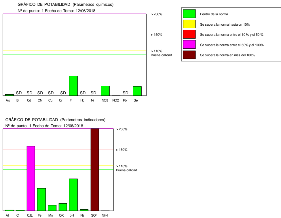
Figura 13. Gráficos de potabilidad del agua de Sondeo Cuesta de las Viñas
