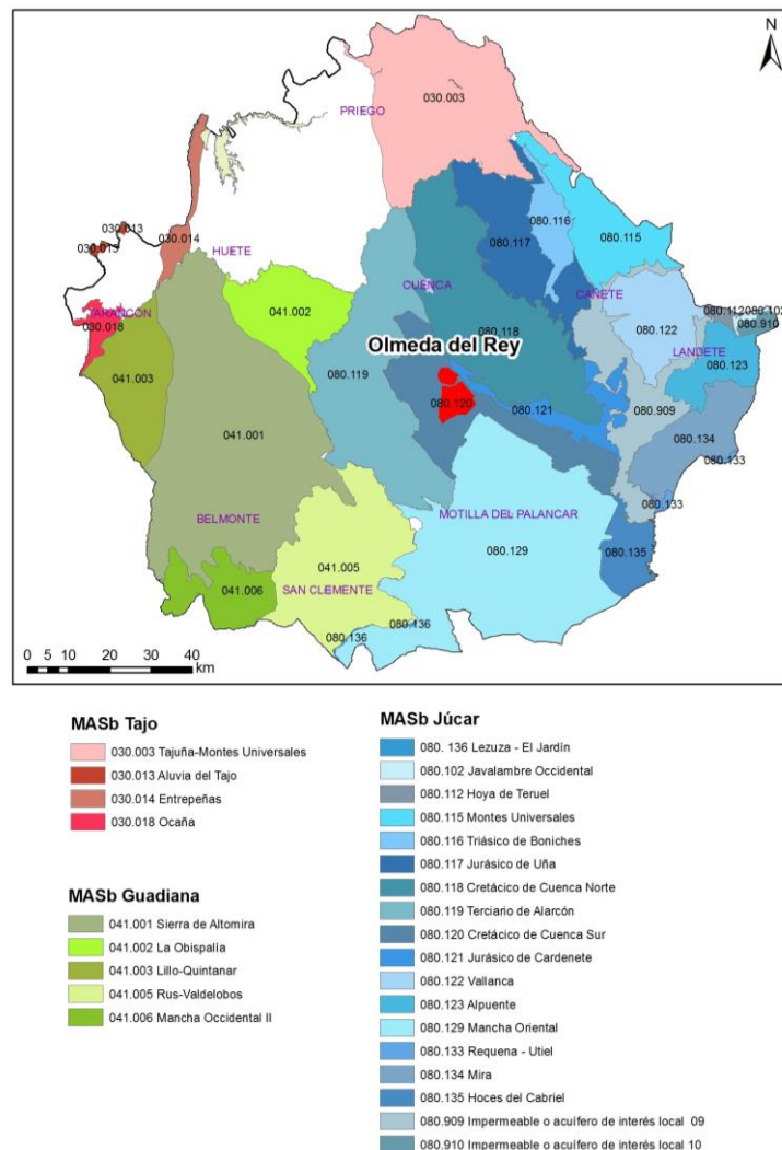
Figura 4. Masas de Agua Subterránea de la provincia de Cuenca y ubicación de Olmeda del Rey
