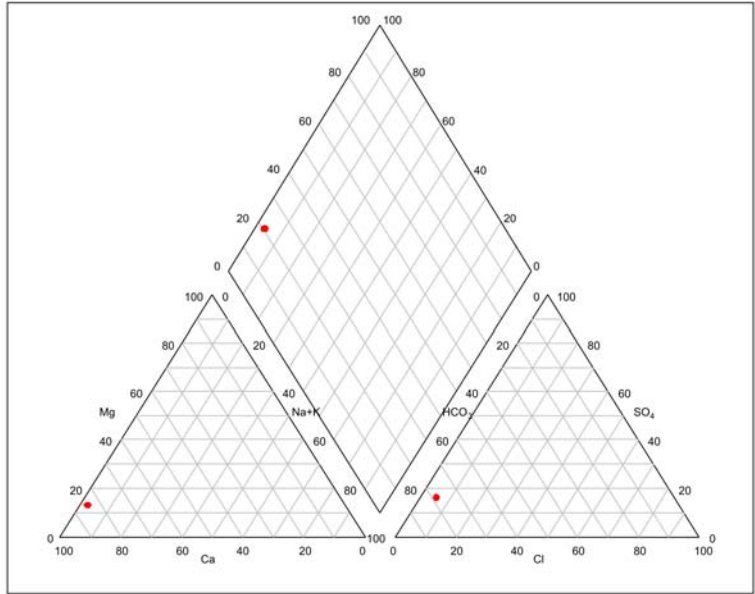
Diagrama de Piper ● Villaseca Manantial 1*
