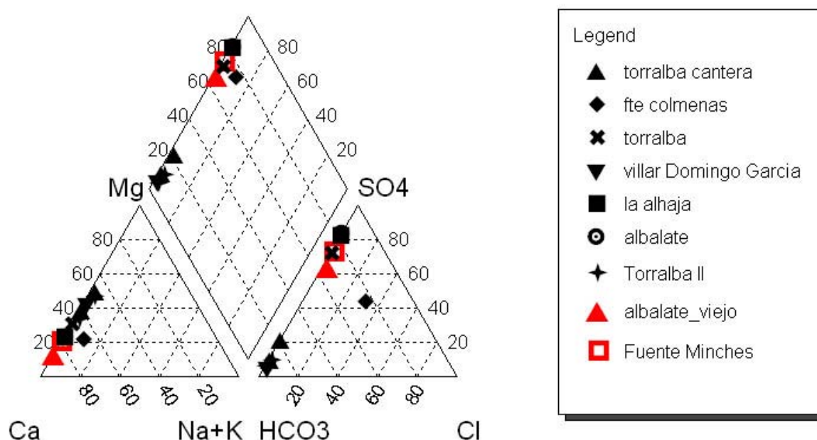
Figura 3- Diagrama de Piper-Hill-Langelier con la representación de las aguas estudiadas.
