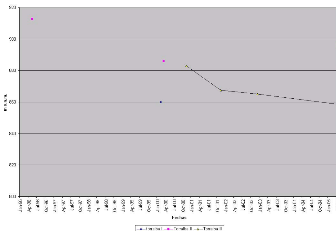
Figura 2. Evolución piezométrica de los sondeos de Torralba, sitios en el flanco occidental de la Sierra de Bascuñana.
