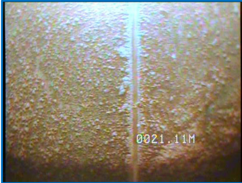
Detalle de ranura, 21,11 m
