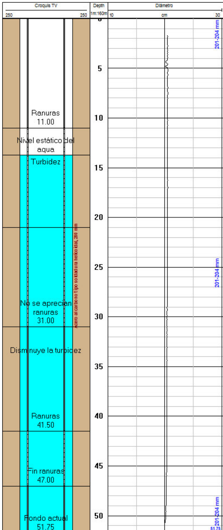
Figura nº 4. Diagrama de diámetros.
