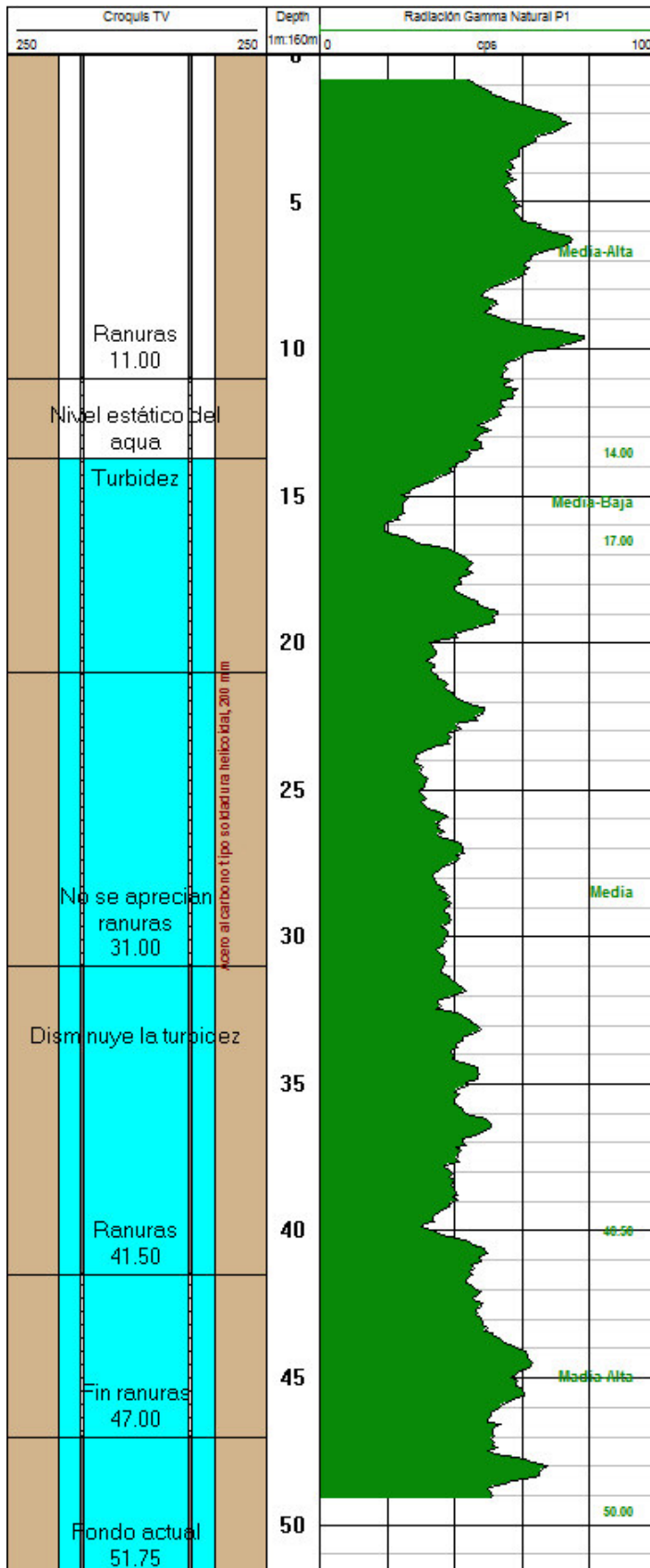
Figura nº 2. Diagrama de radiación gamma natural
