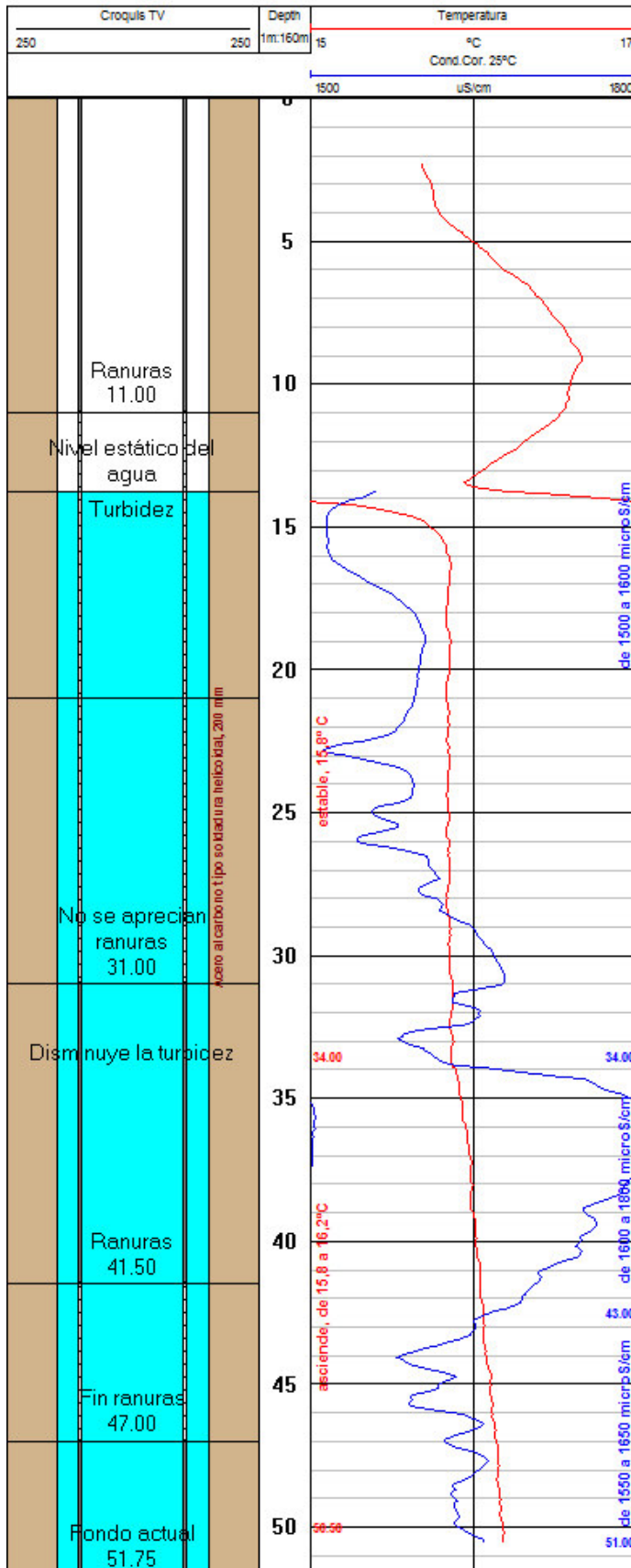
Figura nº 1. Diagrama de temperatura y conductividad.
